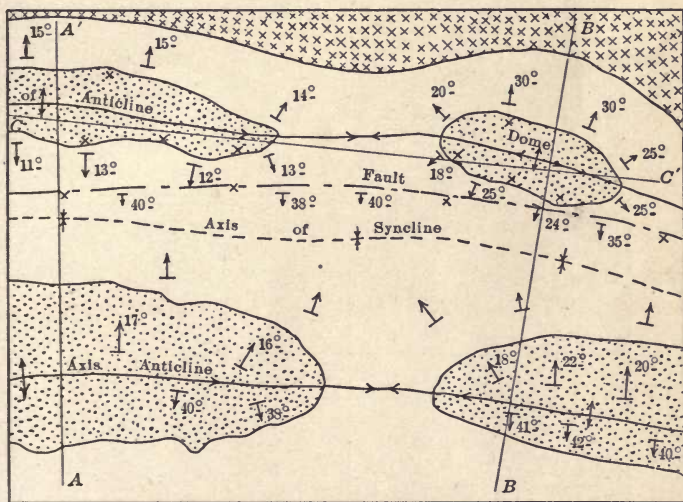
FIG. 31.—Geologic map.
