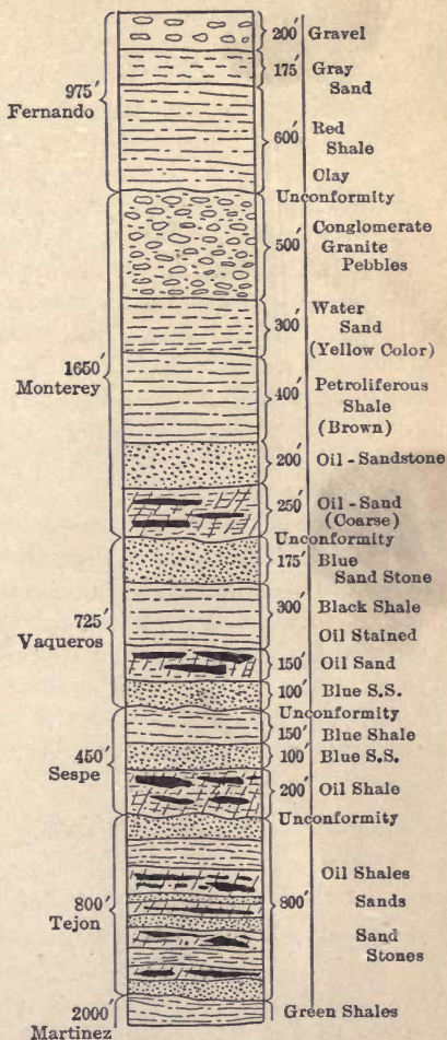
FIG. 7.—Geologic column.
